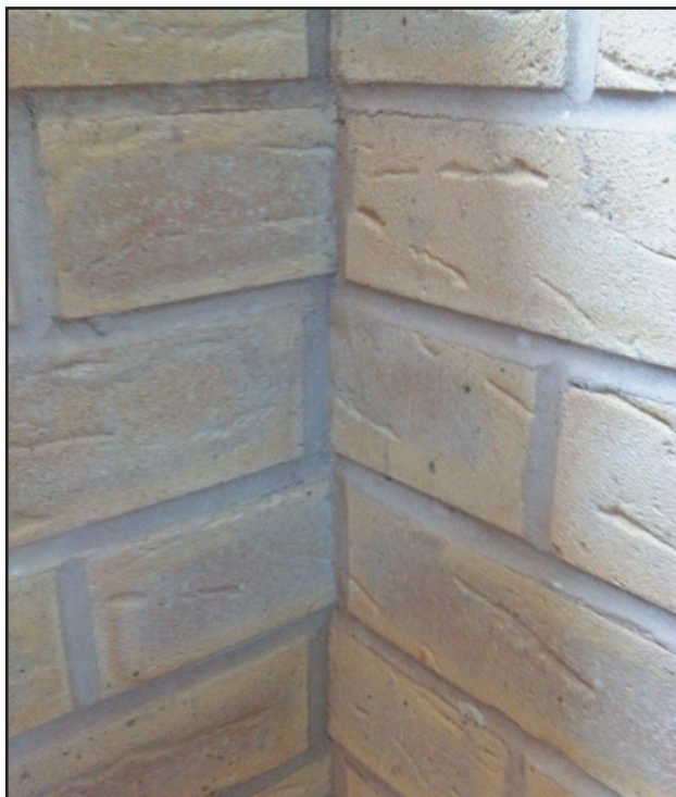
Рис. 165 Правильно выполненный полукруглый шов во внутреннем углу.
