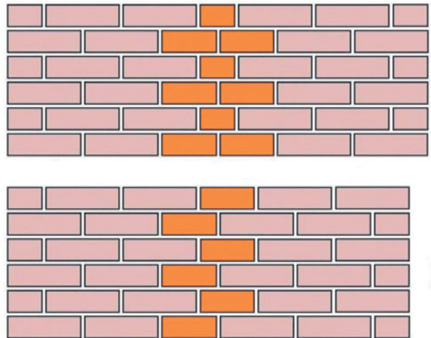
Рис. 100 Примеры ломаной кладки.
