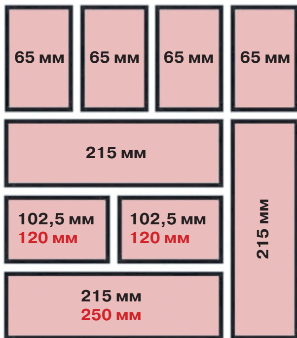
Рис. 26 Согласование размеров кирпичей с учетом 10-миллиметровых швов, заполненных строительным раствором. Красным цветом указаны согласующиеся размеры российского стандартного кирпича.
