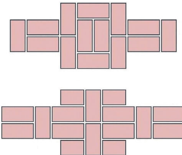
Рис. 202 Фламандская перевязка двойного пилестра шириной в два кирпича (альтернативная схема упрощенной перевязки).
