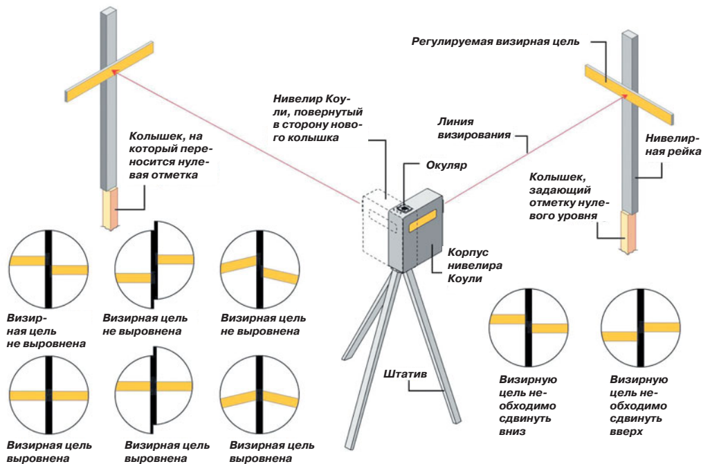
Рис. 59 Порядок работы с нивелиром Коули при переносе высотных отметок.
