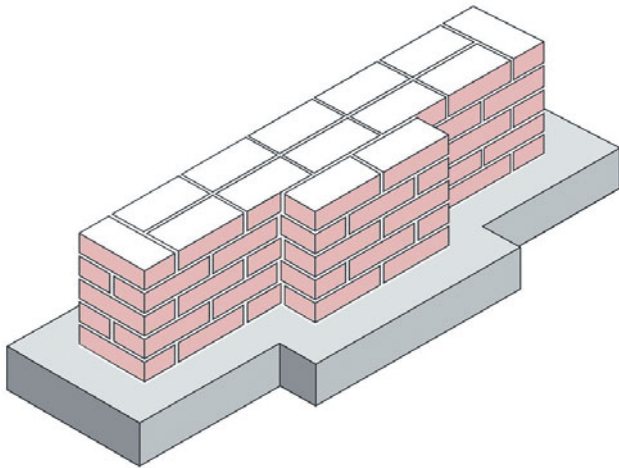
Рис. 40 Ленточный фундамент с выступом внизу и пилястром.
