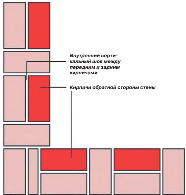
Рис. 94 Кирпичи обратной стороны стены.
