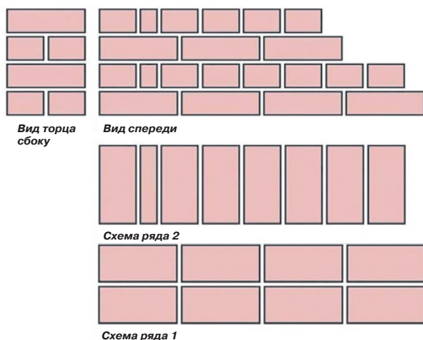
Рис. 89 Английская перевязка.
