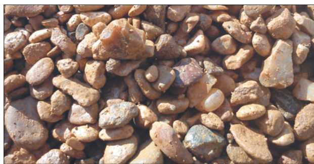
Рис. 4 Крупный заполнитель.
