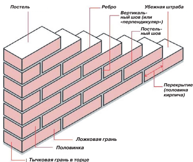
Рис. 83 Термины, используемые при перевязке, и терминология, относящаяся к ложковой перевязке стены.
