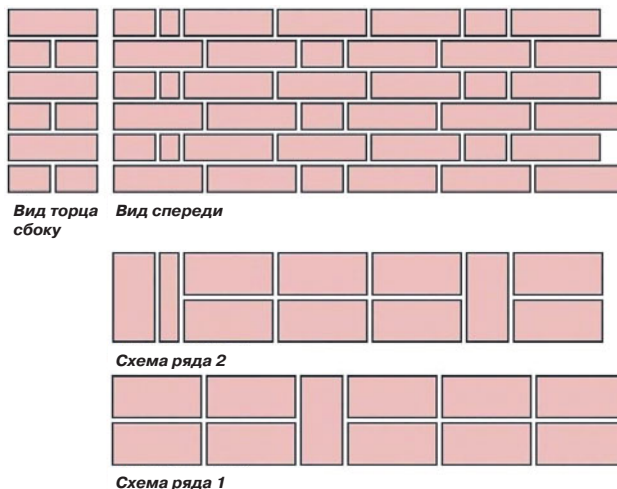
Рис. 98 Фламандская перевязка садовой стены.
