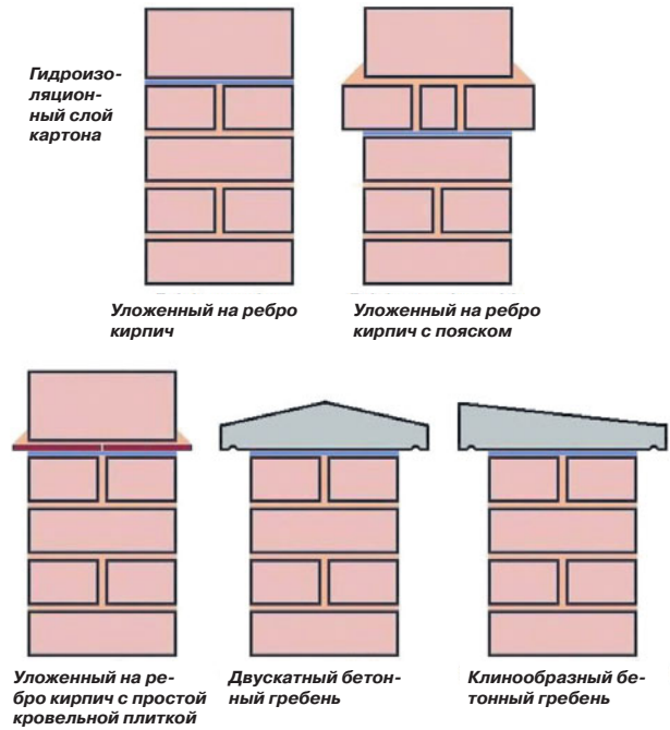
Рис. 208 Простой гребень стены из уложенных на ребро высокопрочных кирпичей.
