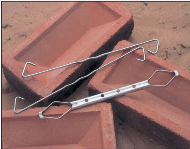
Рис. 170 Современные высококачественные анкеры для пустотелых стен.
