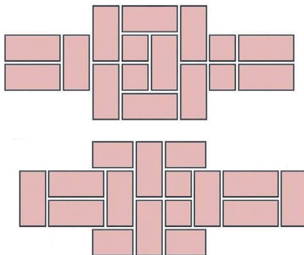
Рис. 201 Фламандская перевязка двойного пилестра шириной в два кирпича.
