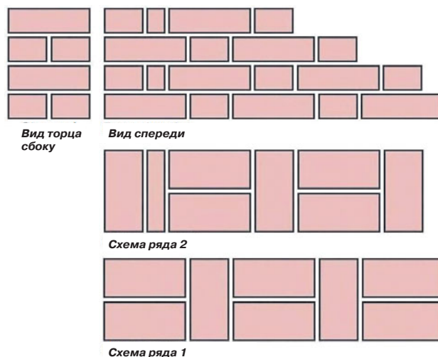
Рис. 90 Фламандская перевязка.
