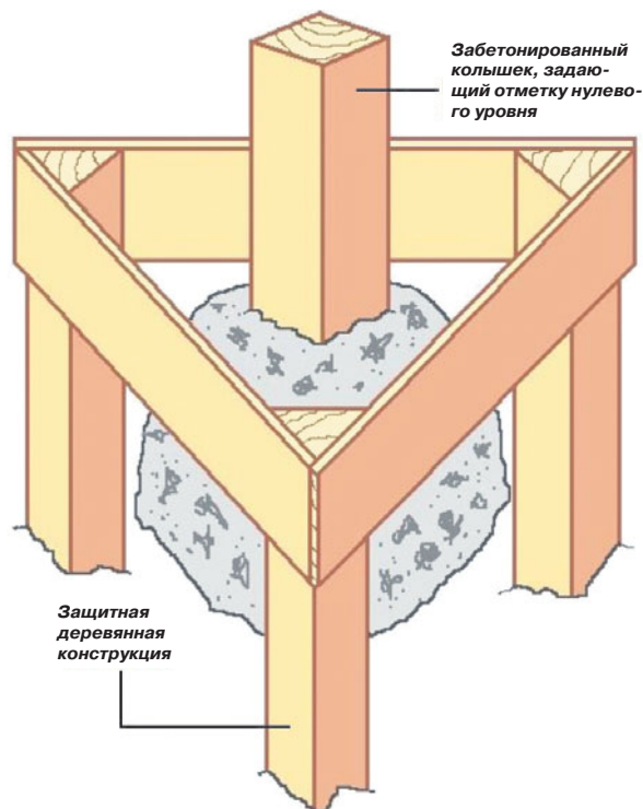
Рис. 56 Забетонированный колышек, задающий отметку нулевого уровня, в защитной деревянной конструкции.
