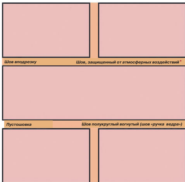
Рис. 153 Стандартные способы расшивки швов.
