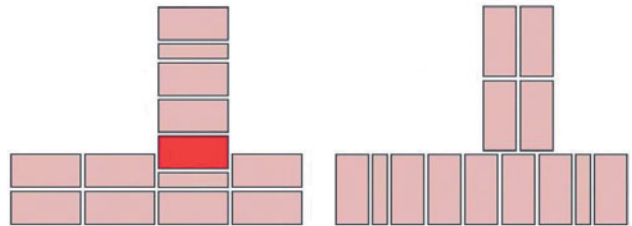
Рис. 95 Английская перевязка примыкающей стены.
