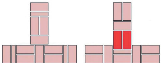
Рис. 96 Фламандская перевязка примыкающей стены.
