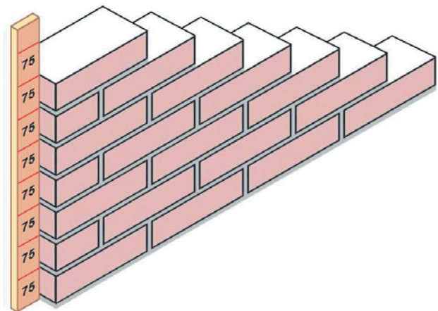
Рис. 124 Контроль кирпичной кладки с использованием порядовки.
