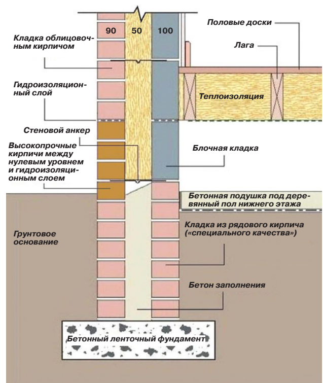
Рис. 167 Пустотелая стена в разрезе; показана типовая конструкция и минимальные размеры в миллиметрах.
