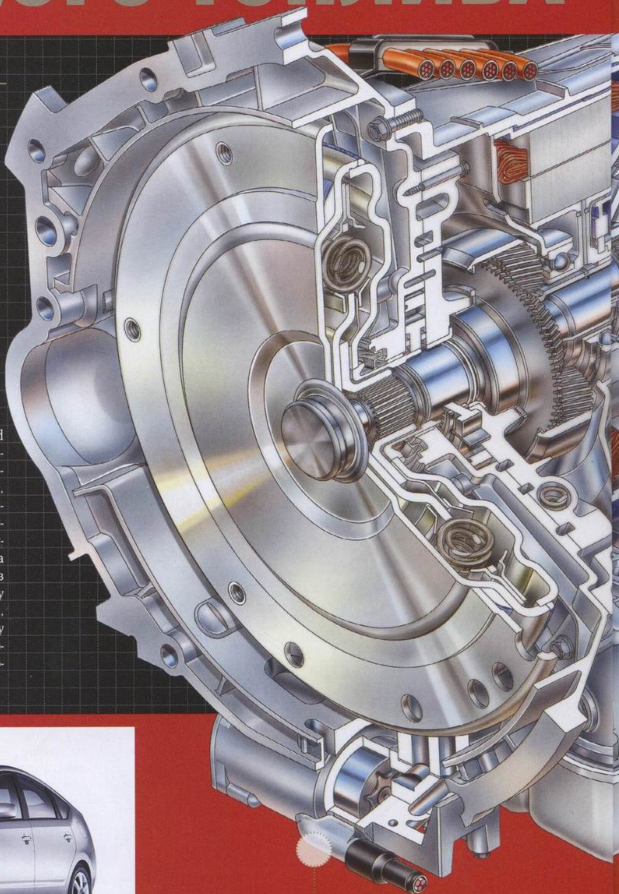
Гибридная силовая установка в версии концерна Daimler Chrysler
