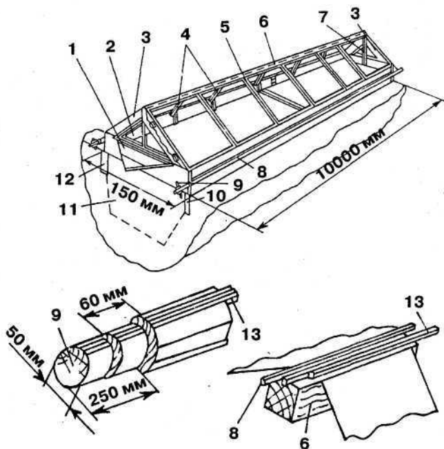
Рис. 6. Цельнодеревянный каркас под пленку: 1 — крышка люка; 2 — вентиляционный люк; 3 — торцы каркаса; 4 — бортовые стойки; 5 — несущие планки; 6 — стропильный коньковый брусок; 7 — бортовая и коньковая стойка; 8 — бобина; 9 — вороток; 10 — правый парубень; 11 — котлован парника; 12 — левый парубень; 13 — рейки-штапики
