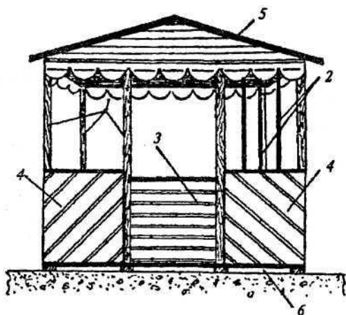
Рис. 2. Вариант устройства незастекленной беседки:
