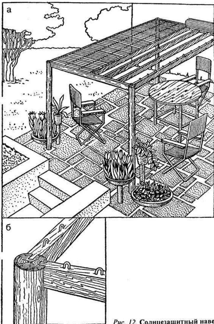
Рис. 12. Солнцезащитный навес
