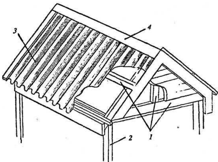
Рис. 4. Конструкция двускатной крыши беседки:
