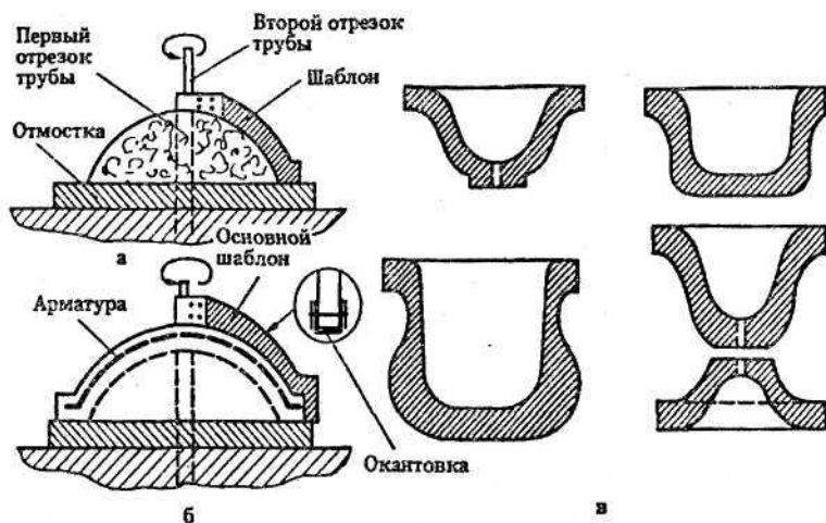
Рис. 15. Технология изготовления железобетонных вазонов
