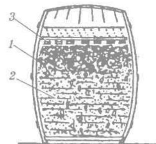
Рис. 4. Брожение в бочке с погруженной шапкой мезги: 1 — мезга; 2 — бродящее вино; 3 — деревянная решетка (шаг реек 1—2 см)
