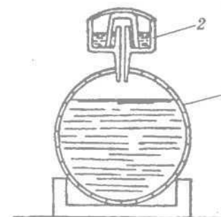
Рис. 2. Бродильный шпунт, установленный в шпунтовое отверстие бочки: 1 — бочка деревянная; 2 — шпунт (затвор)
